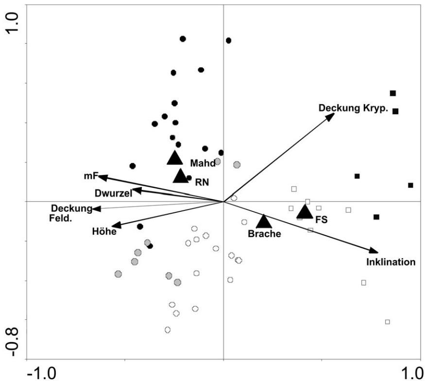
Abb. 3: DCA: Biplot mit allen Vegetationsaufnahmen (n = 54) und Overlay ausgewählter Umweltparameter ( r > 0,4 ; vgl. Tab. 3). Subassoziation von Achillea millefolium , Variante von Rhytidiadelphus squarrosus (●), Typische Variante (◐) und Variante von Scleranthus polycarpus (○); Subassoziation von Viola arvensis , Typische Variante (□) und Variante von Cladonia rangiformis (■). Abkürzungen s. Tab. 3.
